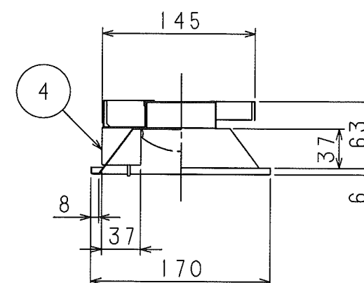
側面詳細図
