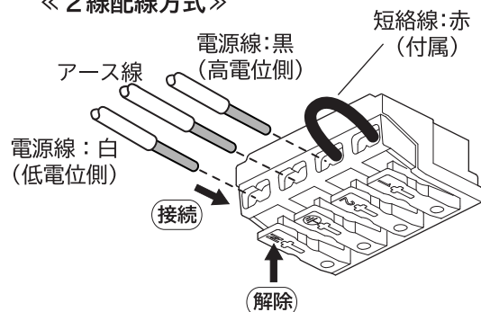
電源端子台の接続と解除(図2)
