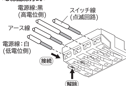
《3線配線方式》
