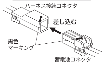
蓄電池コネクタの接続(図3)
