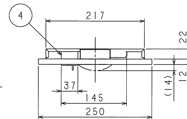
側面詳細図
