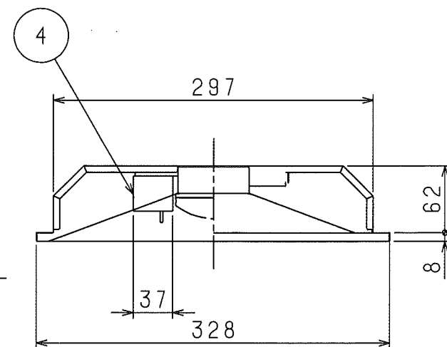
側面詳細図
