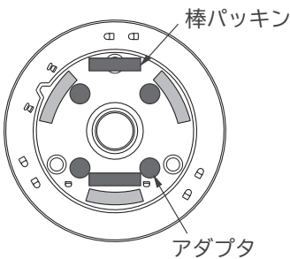
アダプタ
