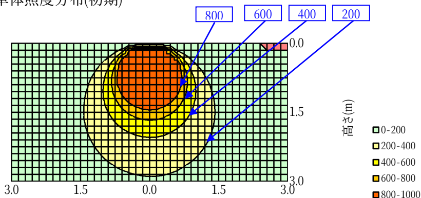
単体照度分布(初期)
