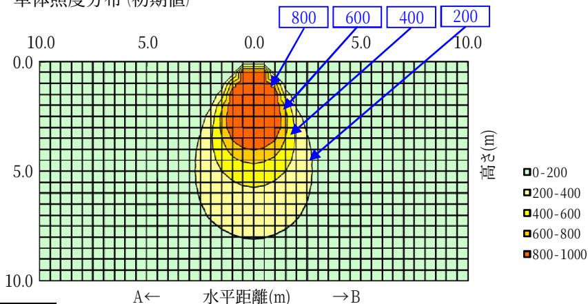
配光曲線 (cd/1000 lm)
