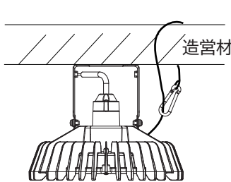
図3 落下防止ワイヤーの取り付け
