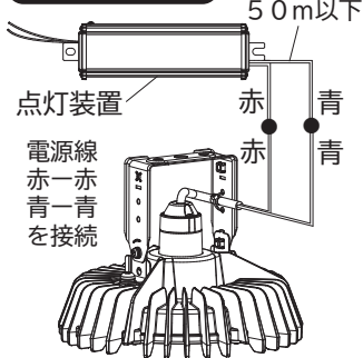
図4 配線接続
