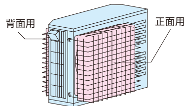
PN-SP10シリーズ 金網ピッチ 50×50mm
