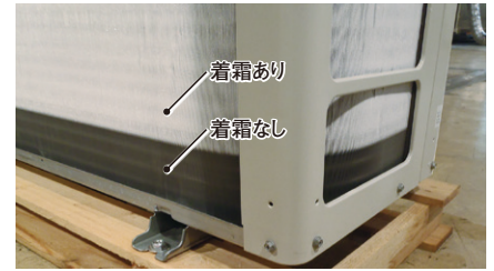
外気温度2℃DB / 1℃CWBの暖房運転時。 製造元の試験室で撮影。
